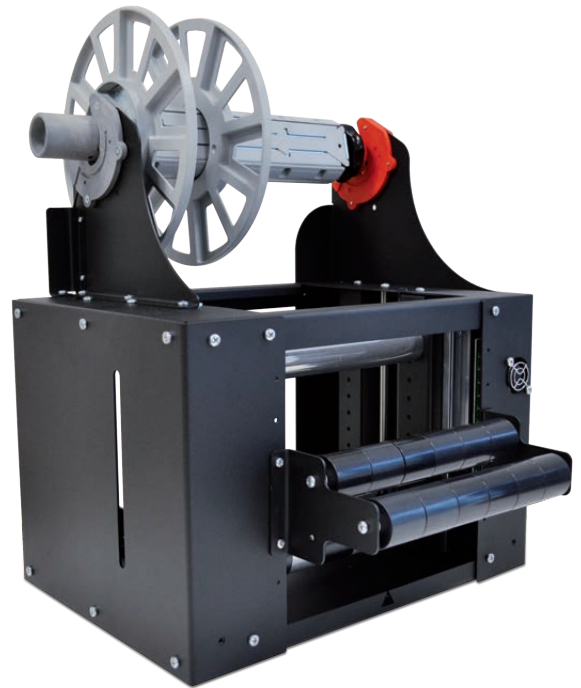
modello MCH100RUXL Avvolgitore MCH XL Velocità 100rpm
